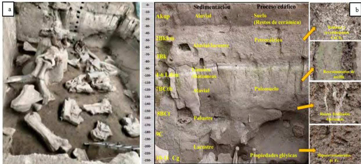
Figura 1 a) Depósito arqueo-paleontológico de San Miguel Tocuila, Texcoco, México b) Estratigrafía y horizontes genéticos y de diagnóstico en el Yacimiento Paleontológico de Tocuila, municipio de Texcoco, Edo. de México.
