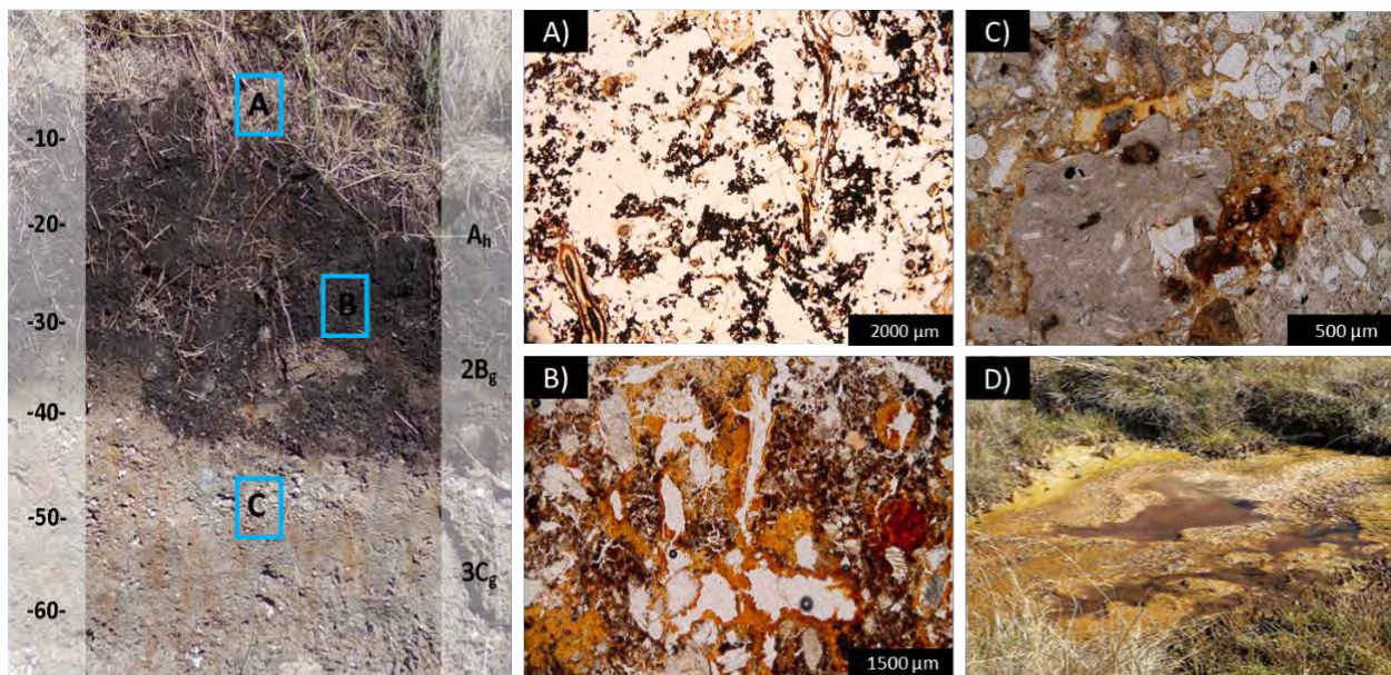
Figura 1. Perfil 1, se observan los rasgos redoximórficos en 2B g y 3C g . A) Estructura migajosa en A h . B) Presencia de hiporevestimientos de (hidr)óxidos de Fe en los poros canal en 2B g . C) Rasgos de empobrecimiento en matriz apedal compuesta de numerosos fragmentos de roca en 3C g . D) Condiciones pobres de drenaje.
