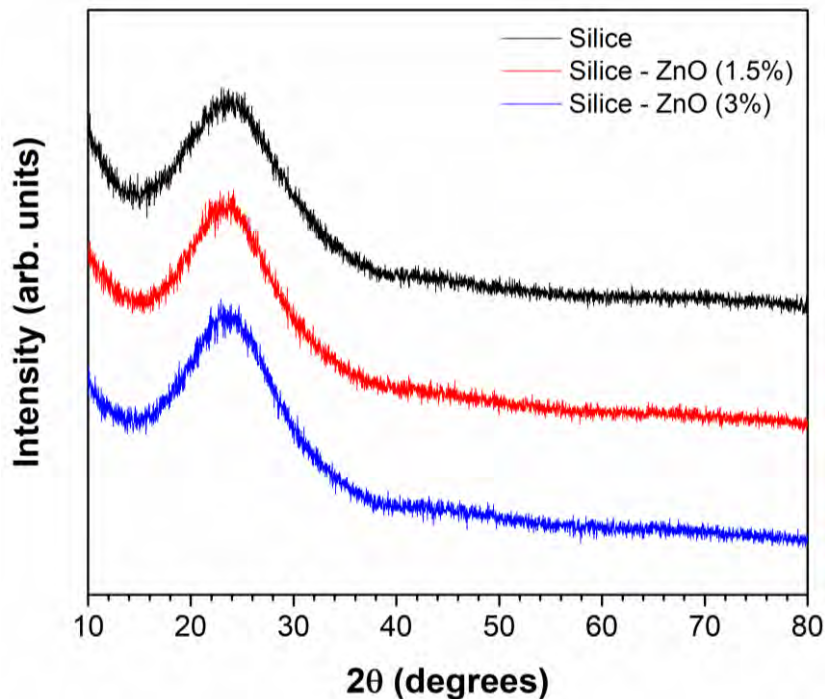
Figura 1. Patrón de difracción de rayos X de nanopartículas de \text{SiO}_2 y \text{SiO}_2\text{-ZnO} .
