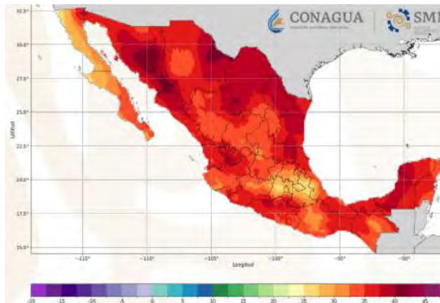
Fig. 1. Comportamiento de las temperaturas máximas durante junio de 2023 (CGSMN, 2023).
